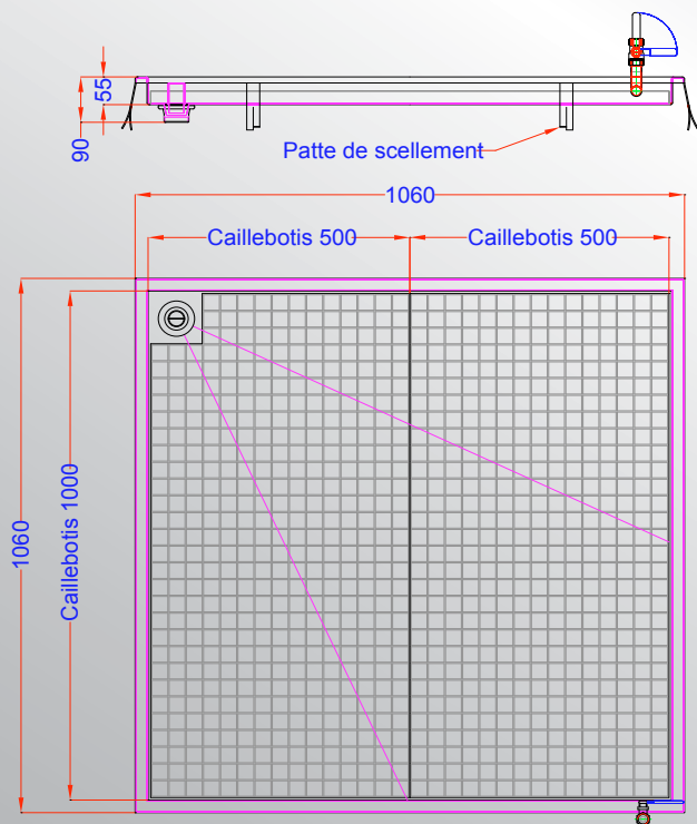
PEDILUVE STANDARD 1000x1000 utiles à encastrer avec vanne d'arrivée (en option)
