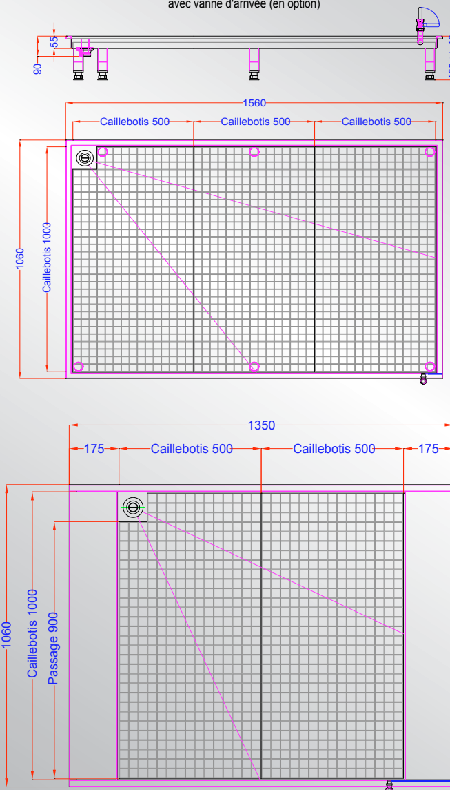
PEDILUVE STANDARD 1500x1000 utiles sur pieds avec vanne d'arrivée (en option)
